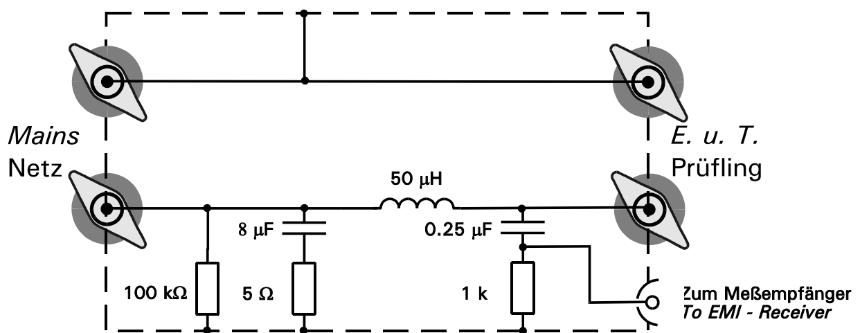
Stromlaufplan (schematisch)
